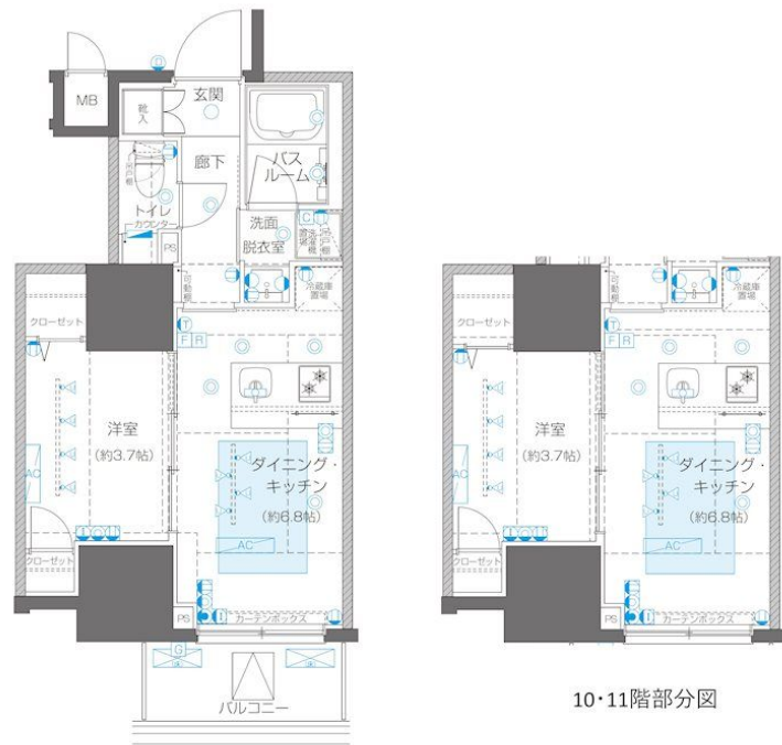
【間取り図】
