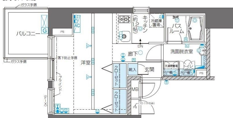
ZOOM目黒/平面詳細図/Fタイプ
