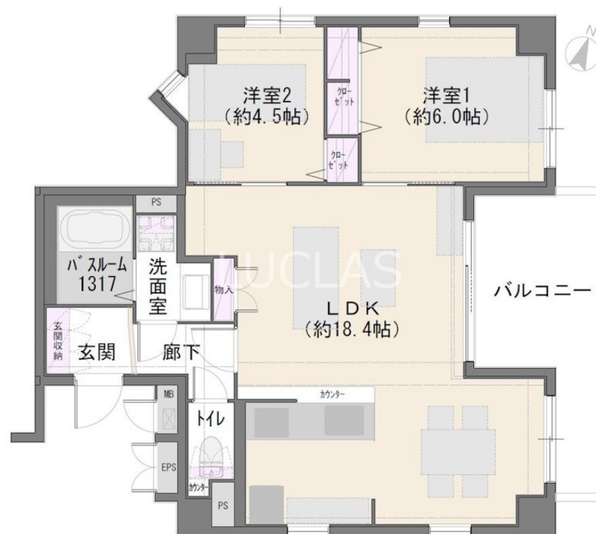
【間取り図】
